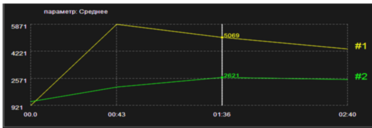
Рис.16. Кривые интенсивность/время в аорте ROI#1 и очаге ROI#2.
