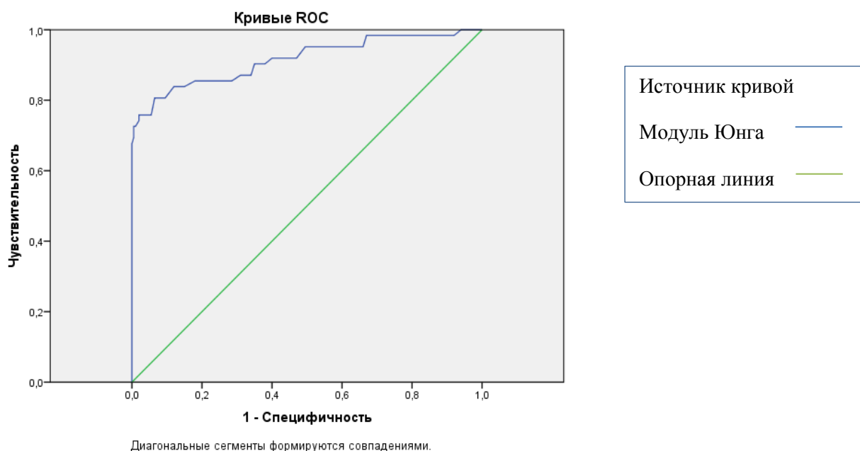
Рисунок 22 – ROC-кривая чувствительности и специфичности значения модуля Юнга у пациентов с хроническими заболеваниями печени
