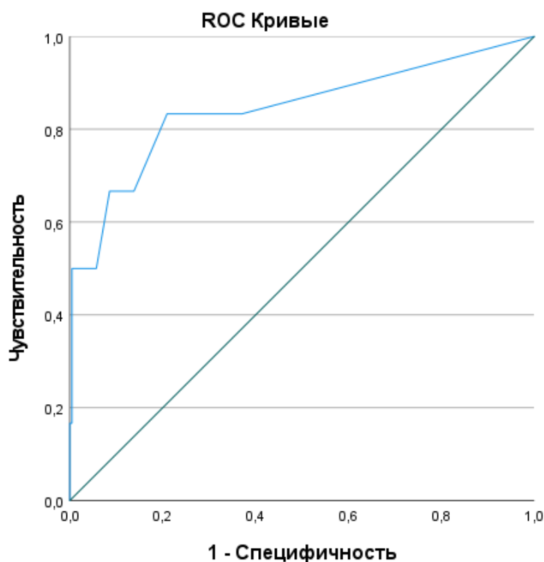
Рисунок 9. ROC - кривая количества метастатических лимфатических узлов центральной зоны при прогнозировании выявления йод-позитивных очагов после радиойодтерапии. По оси абсцисс: 1 - специфичность (доля ложноположительных результатов); по оси ординат - чувствительность (доля истинно положительных результатов). Диагональная линия соответствует тесту, не имеющему диагностической ценности ( AUC = 0,5 ).
