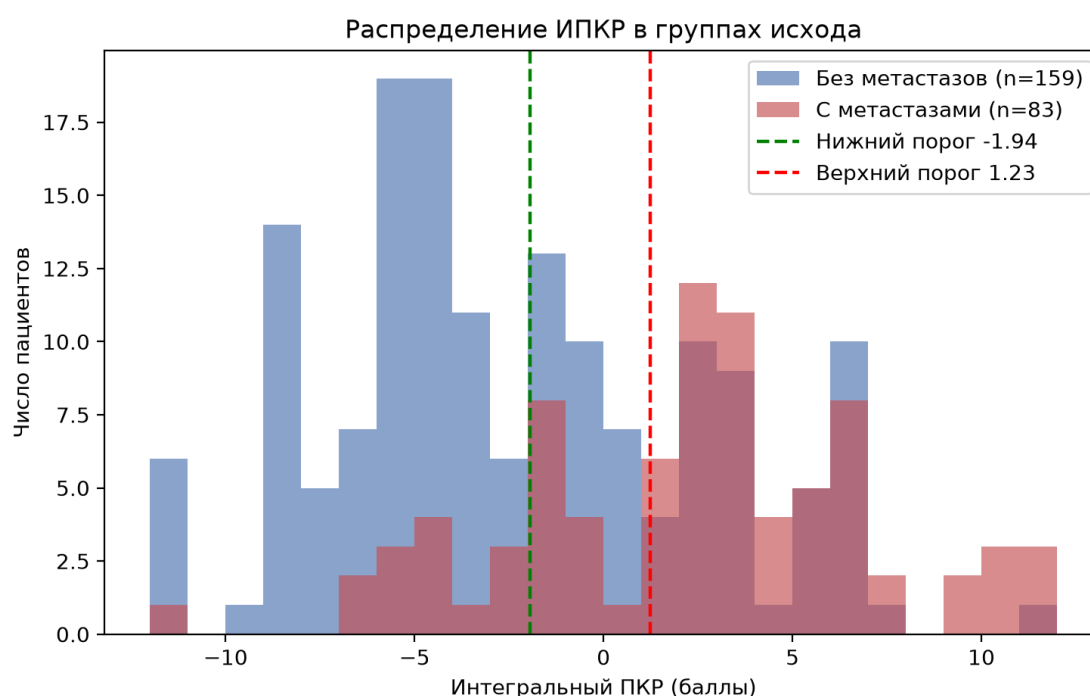
Рисунок 4. Распределение интегрального ПКР в группах сравнения (с и без метастазирования).
