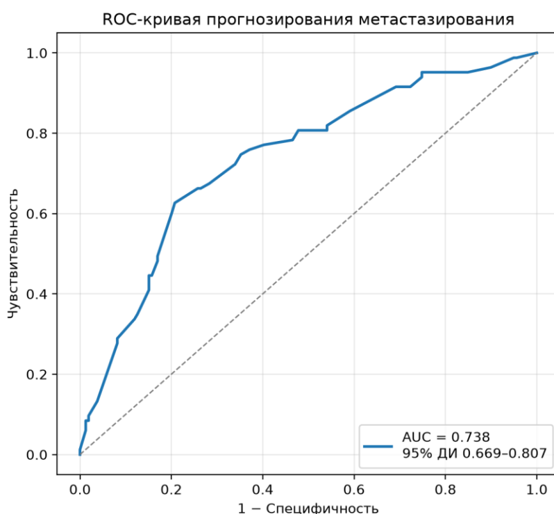
Рисунок 5. ROC-кривая прогнозирования метастазирования в ЛУ центральной зоны. По оси абсцисс - 1 - специфичность (доля ложноположительных результатов); по оси ординат - чувствительность (доля истинно положительных результатов). Диагональная линия соответствует тесту, не имеющему диагностической ценности (AUC = 0,5).
