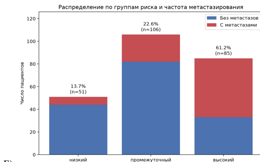
Рисунок 6. Распределение интегрального ПКР и групп риска. А) Распределение ИПКР в группах исхода (с метастазами и без); пунктирные линии - эмпирические пороги (-3,98 и +1,41). Б) Распределение пациентов по группам риска и наблюдаемая частота выявленного метастазирования
