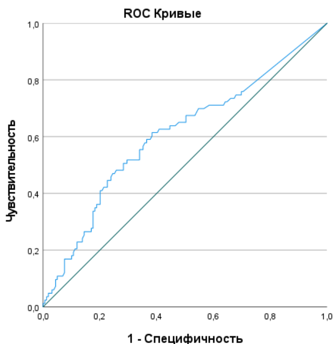
Рисунок 2. ROC-кривая количественной представленности мутации BRAF V600E при прогнозировании метастазирования в ЛУ центральной зоны. По оси абсцисс: 1 - специфичность (доля ложноположительных результатов); по оси ординат - чувствительность (доля истинно положительных результатов). Диагональная линия соответствует тесту, не имеющему диагностической ценности ( AUC = 0,5 ).
